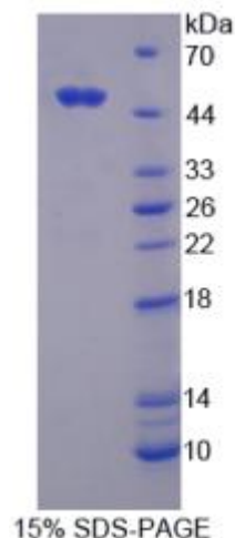
15% SDS-PAGE
