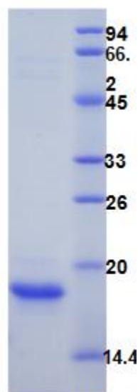
15% SDS-PAGE
